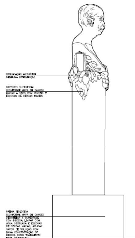
3 | HERMA DE RUI BARBOSA ELEVÇÃO LATERAL ESQUERDA ESC 1:10
