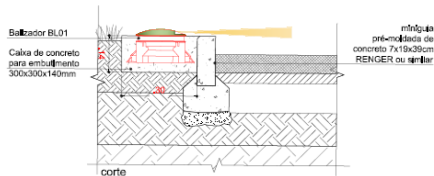
DETALHE CAMINHOS INTERNOS ESCALA 1:10
