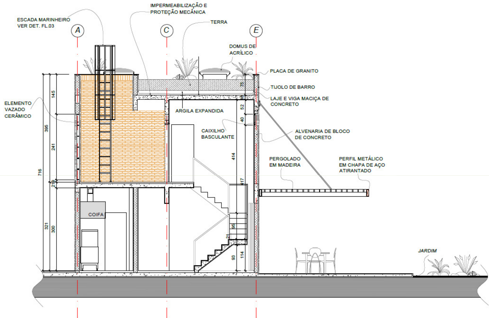
CORTE CC - TRANSVERSAL
