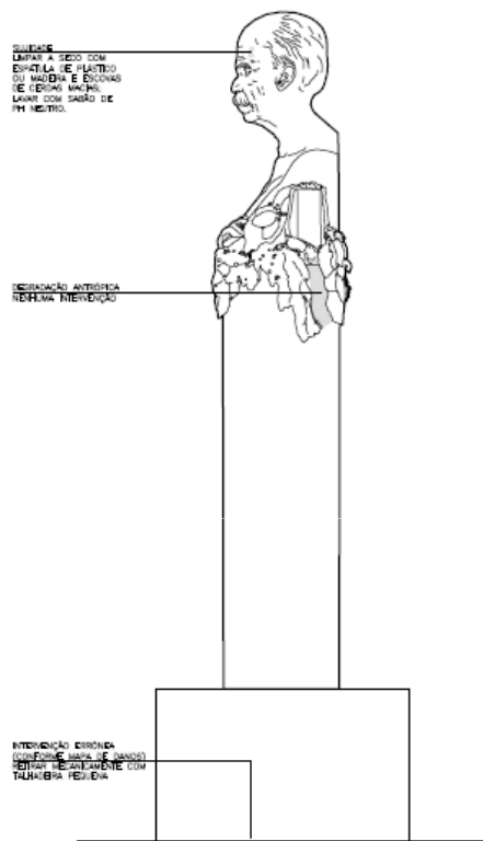
3 | HERMA DE RUI BARBOSA ELEVÇÃO LATERAL DIREITA ESC 1:10
