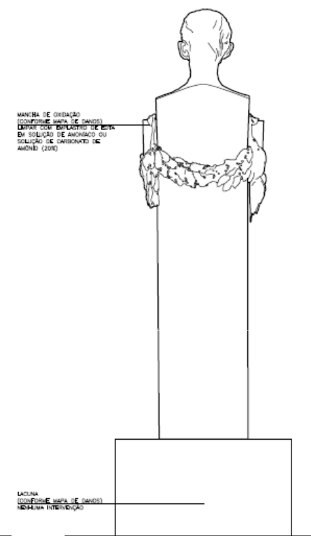
3 | HERMA DE RUI BARBOSA ELEVÇÃO COSTAS ESC 1:10
