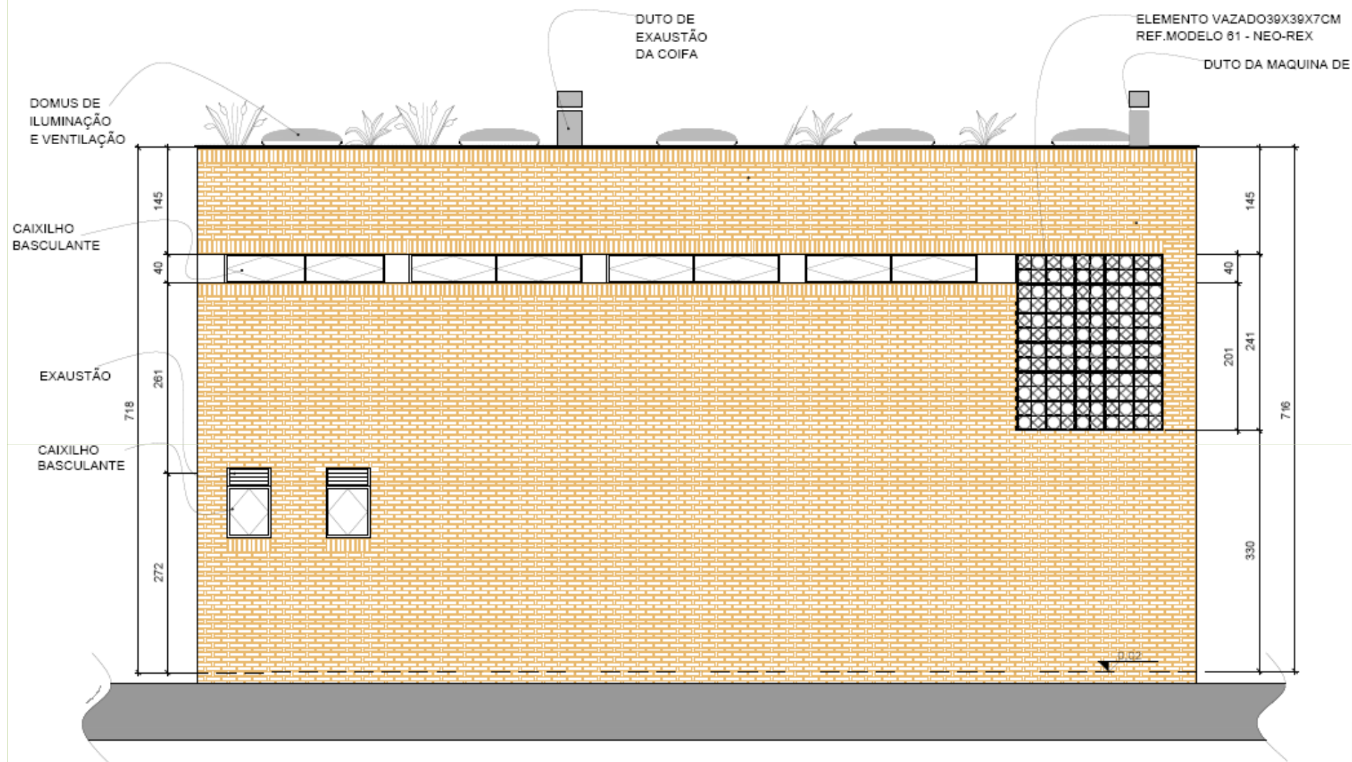
ELEVAÇÃO POSTERIOR
