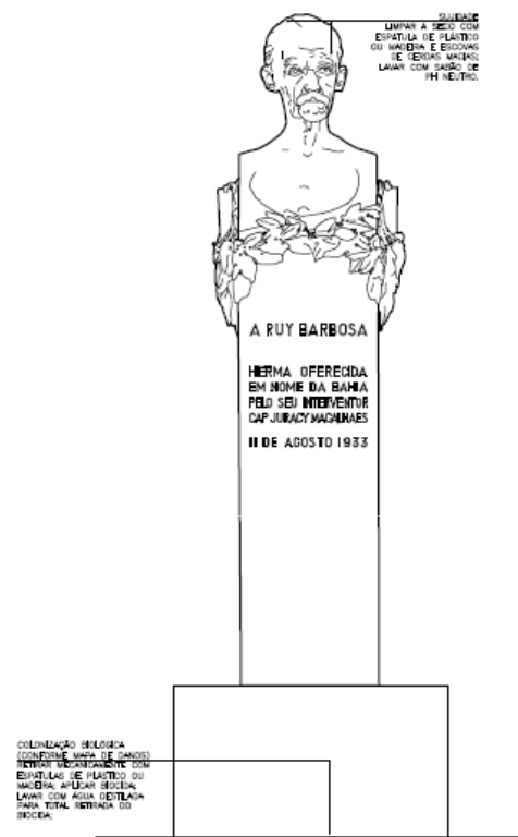
3 | HERMA DE RUI BARBOSA ELEVÇÃO FRONTAL ESC 1:10
