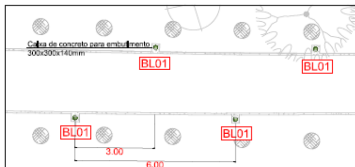
LOCAÇÃO CAMINHOS INTERNOS ESCALA 1:10
